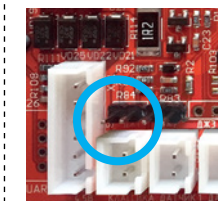
Минимальная чувствительность – перемычка удалена
