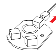
Отсоедините провод от контактной пластины, сильно потянув за провод
