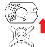
Снимите контактную пластину с основания, подняв ее вверх
