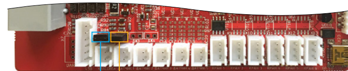
Джемпер №2 – управление силовым энергозависимым реле Джемпер №1 – управление чувствительностью датчиков
